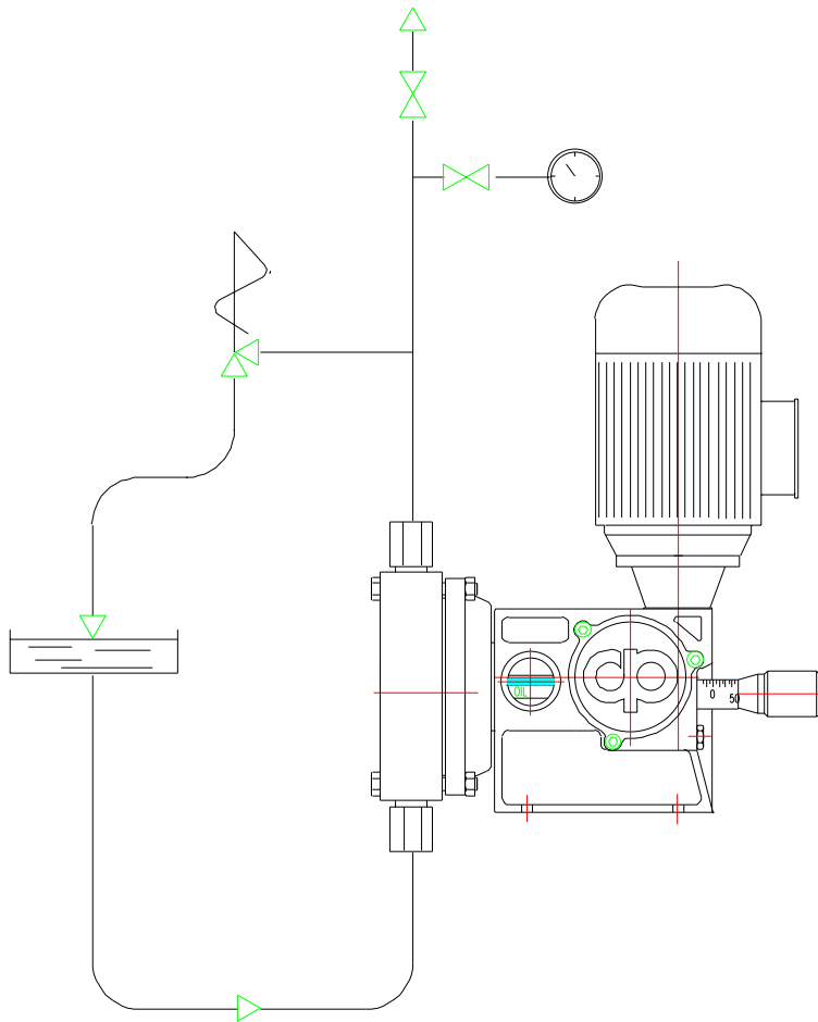
Fig. 07 (installazione di valvola di sicurezza e manometro)
